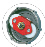
Riduttore a satelliti e planetario (M16)
