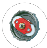
Planetengetriebe
